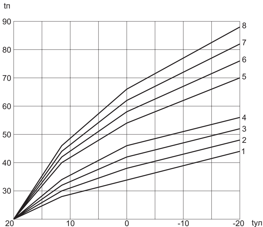
Рис.3.5. Кривые погодозависимой регулировки
