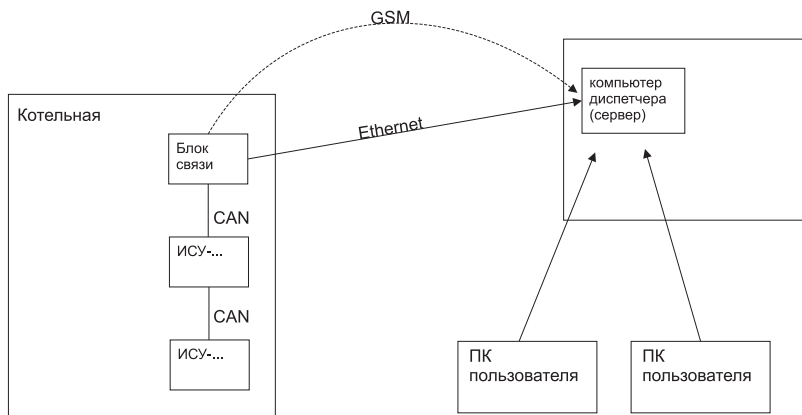
Рис.6.1. Схема построения системы диспетчеризации
