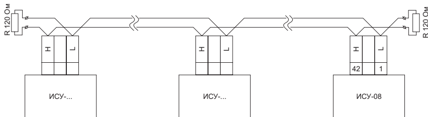
Рис. 2.11. Схема объединения в сеть
