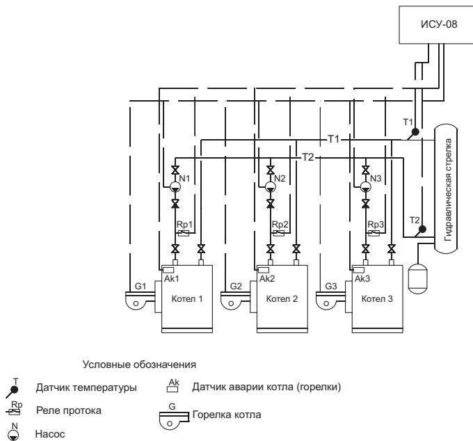
Рис. 2.2. Схема управления котлами
